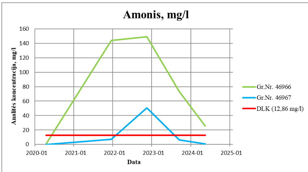
4 pav. Amonio koncentracijos kaita 2020-2024 m. gręžinių Nr. 46966, 46967 vandenyje
